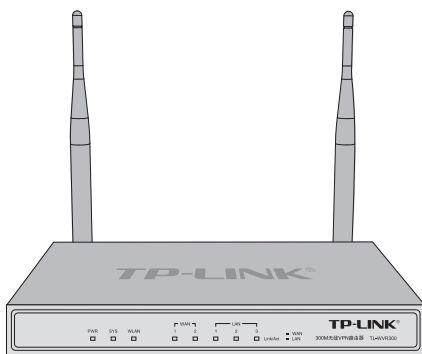
图1-1 TL-WVR300前面板示意图
